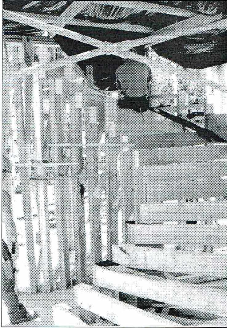
mise en place du fut tracé des marches, remontée par rapports a la vue en plan
